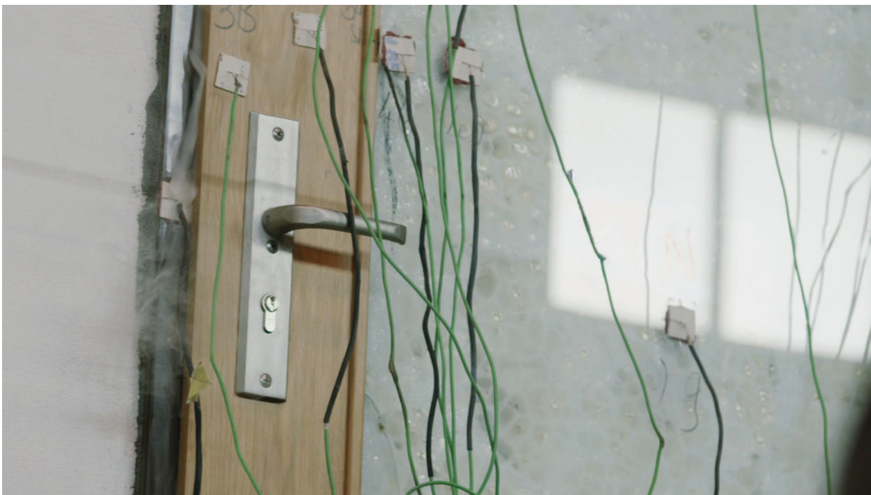
Dveře během požárních zkoušek.
