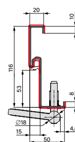
ROHOVÁ OCELOVÁ ZÁRUBEŇ
