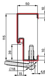
OCELOVÁ ZÁRUBEŇ
