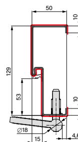
OCELOVÁ ZÁRUBEŇ
