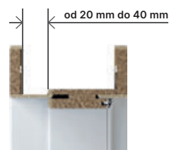
ZÁRUBĚ S PRODLOUŽENÝM PEREM volitelně za příplatek
